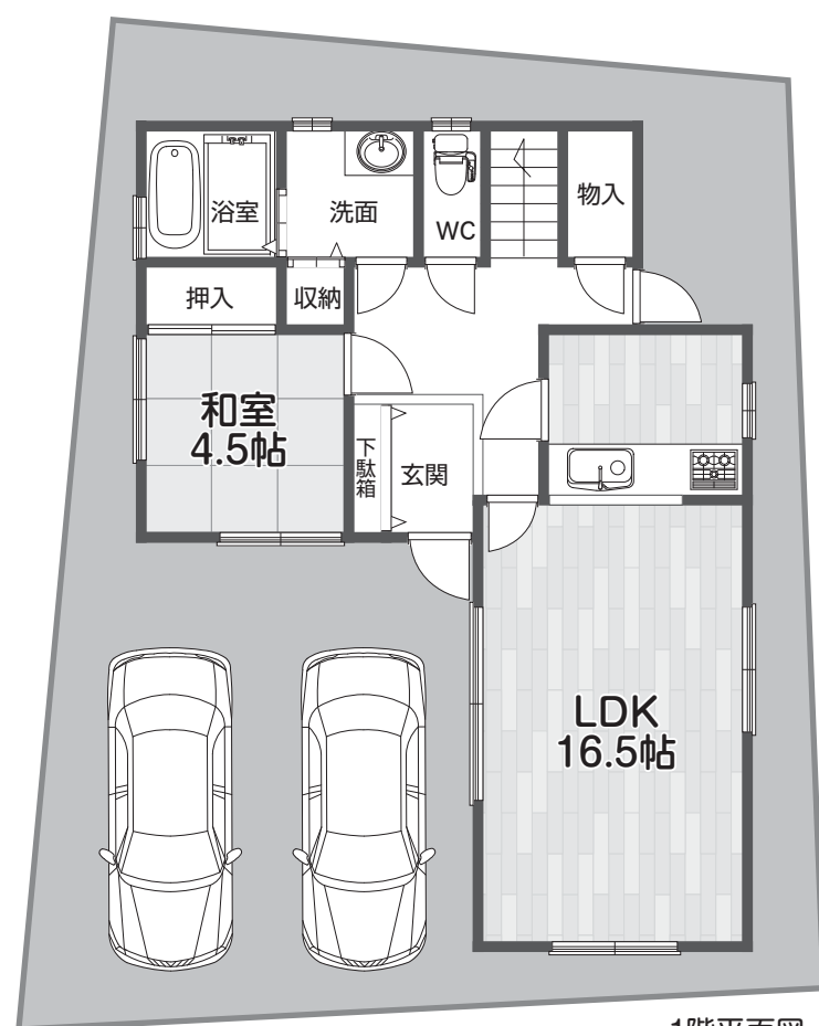
1階平面図
